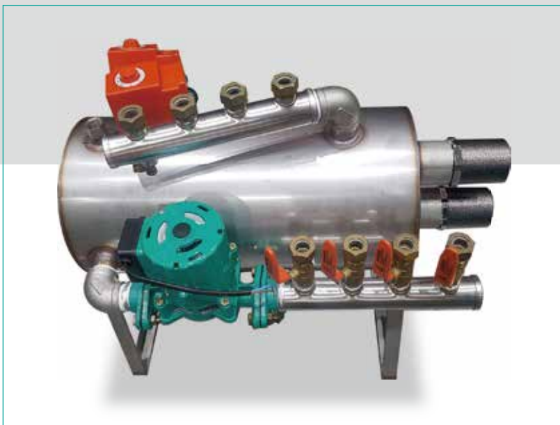
생육실 온수순환기
